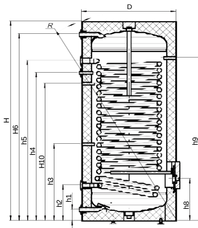
Diagram 1 - Ohříváč vody Triven BTM
