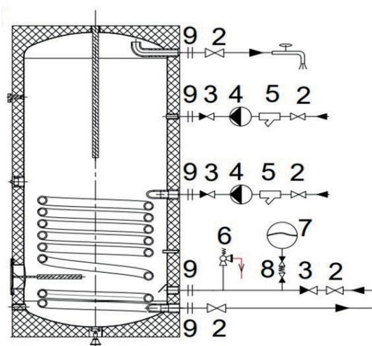
Obrázok 6. Typická odporúčaná schéma zapojenia ohrievača vody
